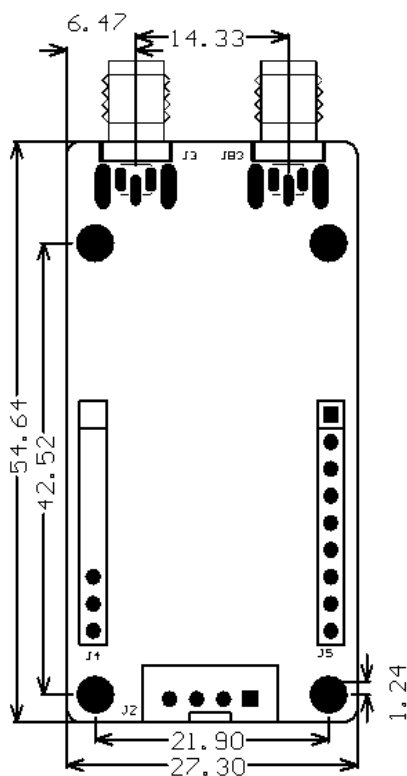
图 1.4 尺寸图
