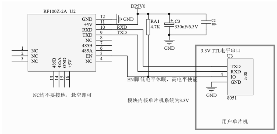
图 1.5 外围电路图
