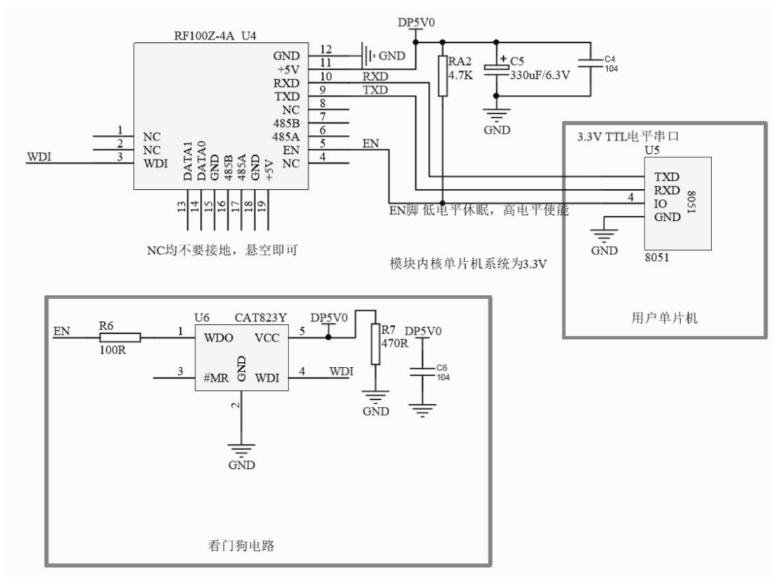
图 1.5 外围电路图
