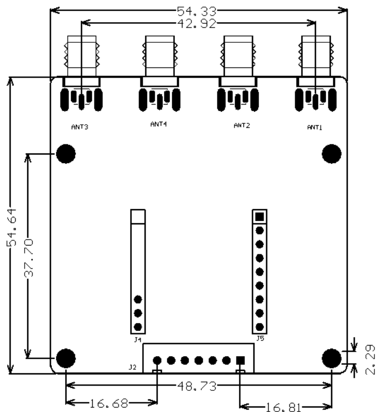
图 1.4 尺寸图
