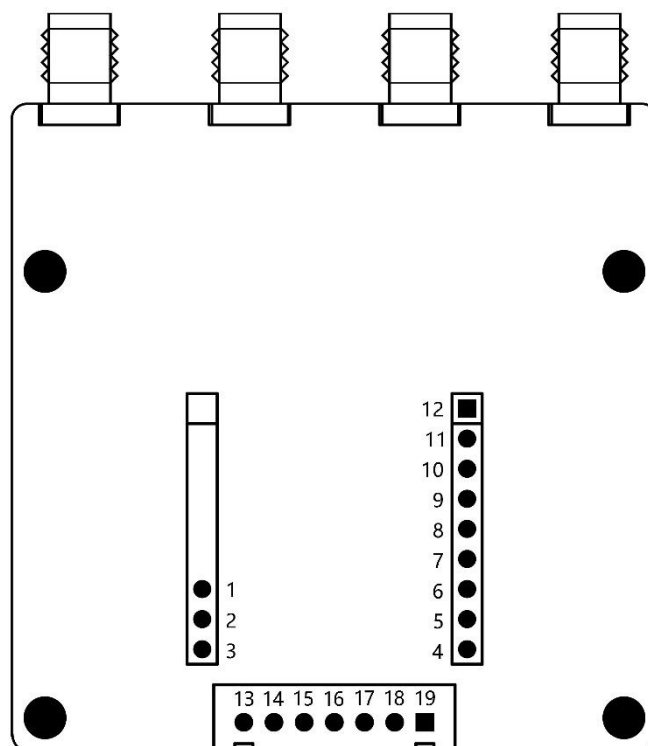
图 1.1 TOP VIEW
