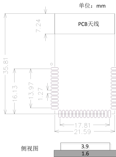
图 1-2 WLT2420SZ 结构尺寸
