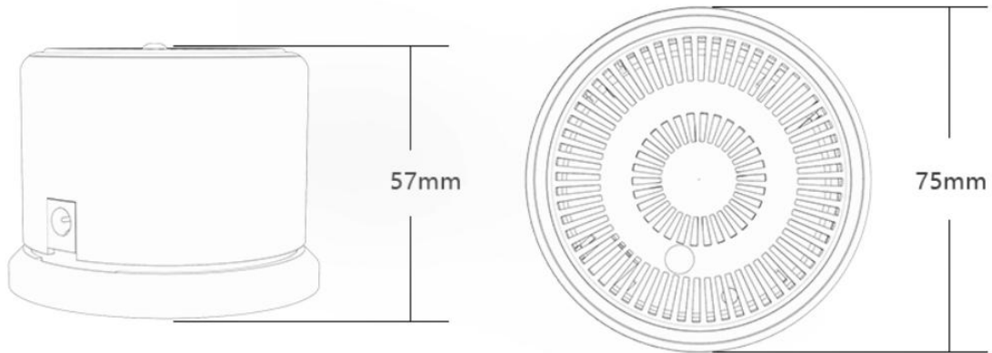
机械尺寸图
