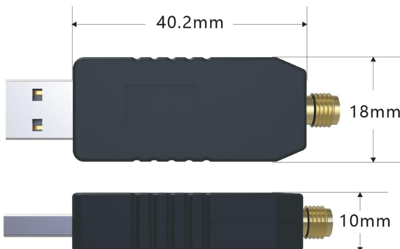
图 1-2 WLT2420NZ-USB 结构尺寸
