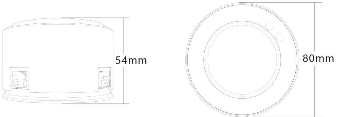
机械尺寸图
