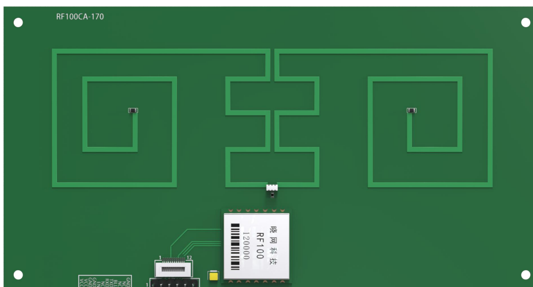
图 1-1 RF100CA-170 近场天线
