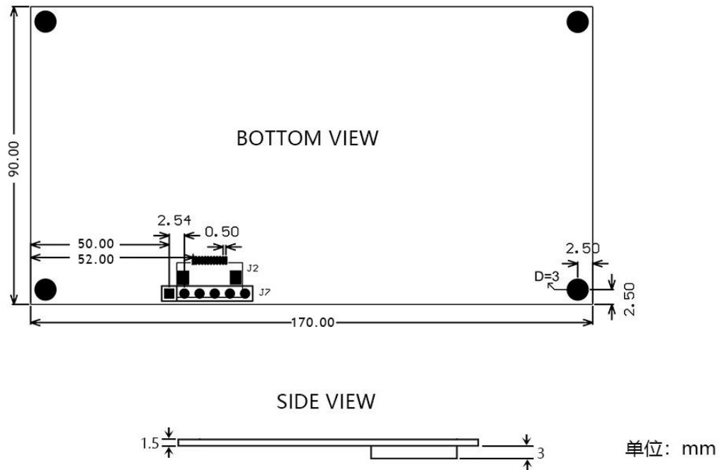
图 1-5 产品尺寸图
