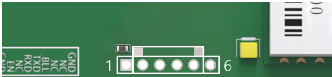
图 1-3 排针线序
