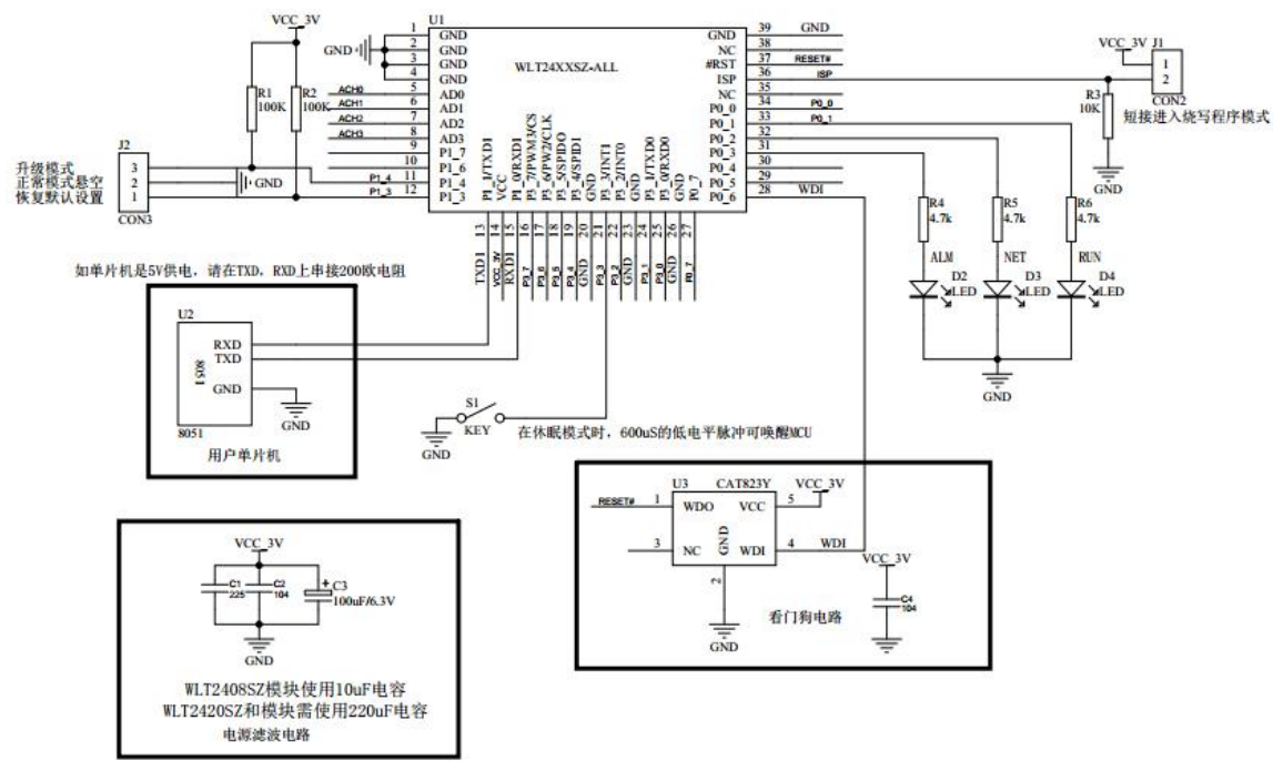
本电路适合的模块为WLT2408SZ和WLT2420SZ
